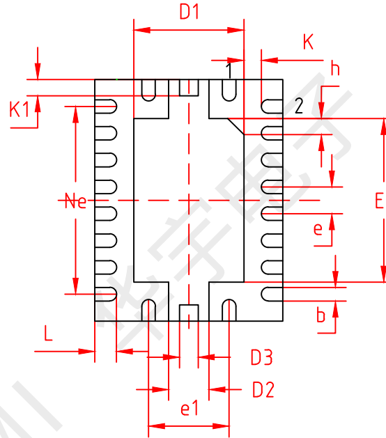
BOTTOM VIEW 背视图
