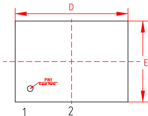
正视图
